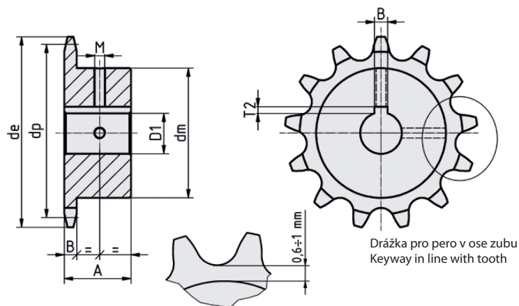
Indukčně kalené zuby HRC 45÷53 Induction hardened teeth HRC 45÷53
